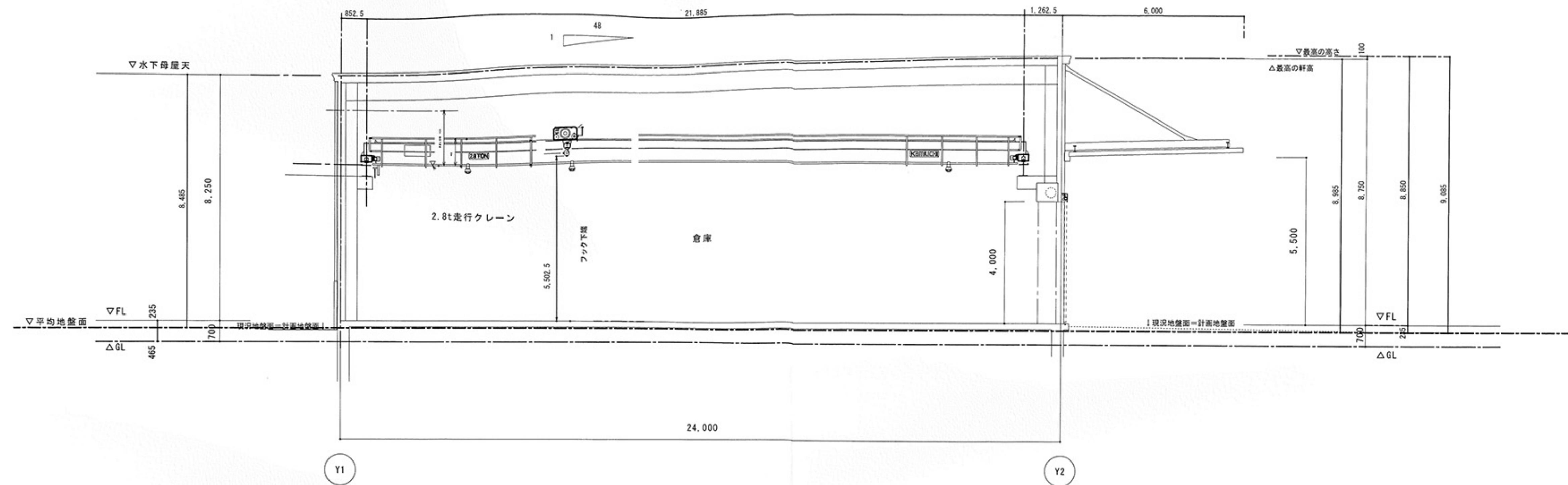
Y方向断面図 S=1/100
