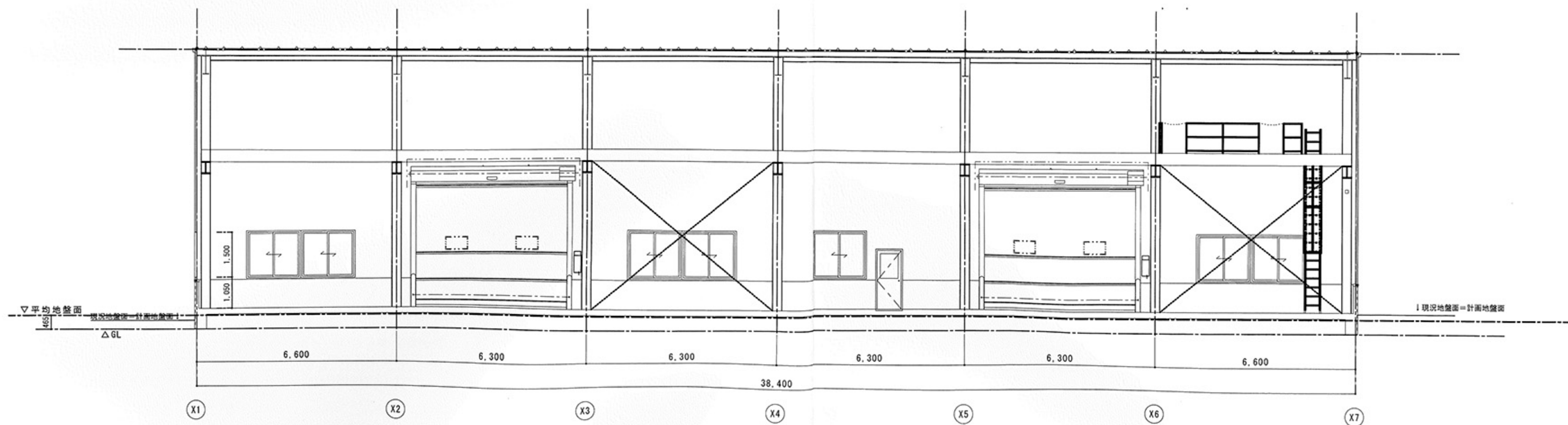
X方向断面図 S=1/100
